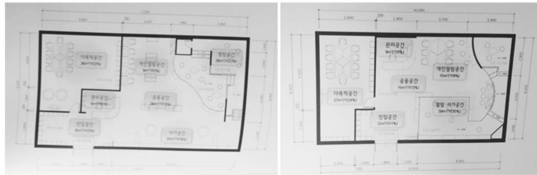
중규모 165㎡ 공간구성
