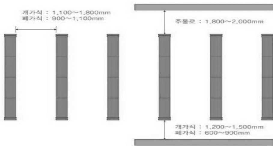
그림 4-3. 서가 배치간격
